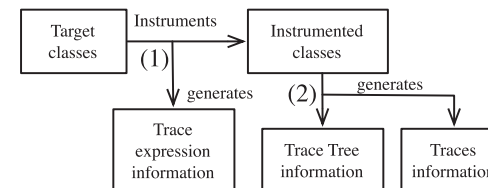
図 7 トレースの記録の行程
