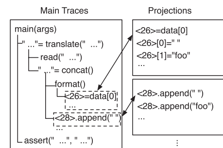
図3 トレースを利用したデバッグにおける追跡のための表示 Fig. 3 Views for navigation of trace based debugging.
