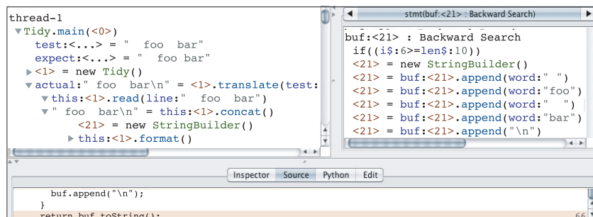
図 5 Traceclasses のトレース表示部分
