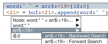
図 6 局所的な追跡のためのトレース表示 (上) と検索のためのメニュー (下)
