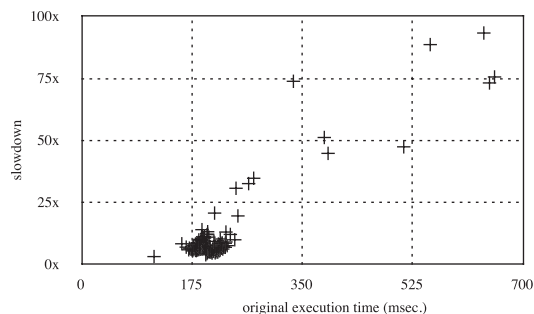
図 10 jtidy の 223 テストケースの本来の実行時間とトレースを記録した場合の速度低下の分布 Fig. 10 Distribution of original execution time of jtidy's 223 test cases and slowdown by recording traces.
