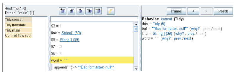
図2 TOD 14) による追跡の例：各表示は、左はメソッド呼び出しスタック、中央は選択されたメソッド内部のトレースのリスト、右は選択されたトレースの時点の状態を表す
